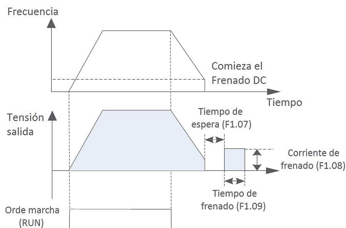
Figura 6-3-6 Rampa desaceleración + Frenado DC
