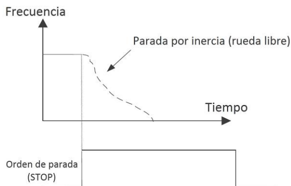
Figura 6-3-5 Parada por inercia (rueda libre)
