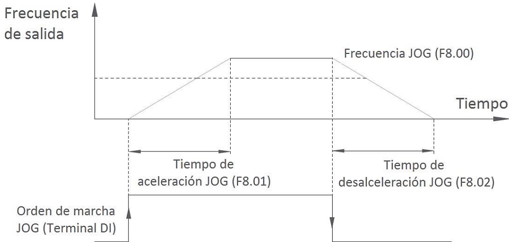
Figura 6-13-1 Función de avance lento (JOG)
