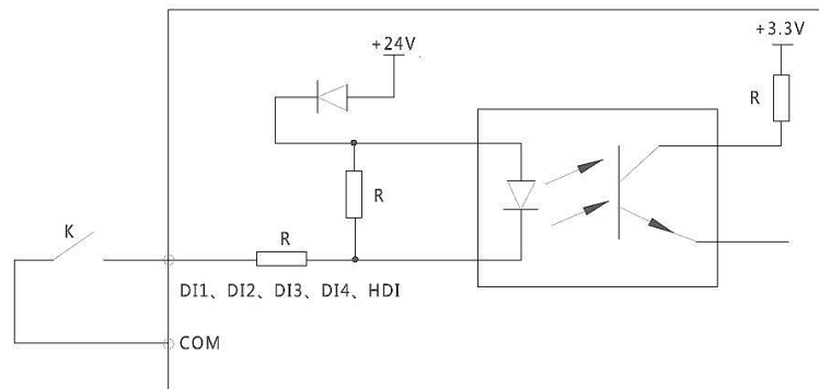
Figura 3-6-1 Entradas DI Esquema de conexión interna
