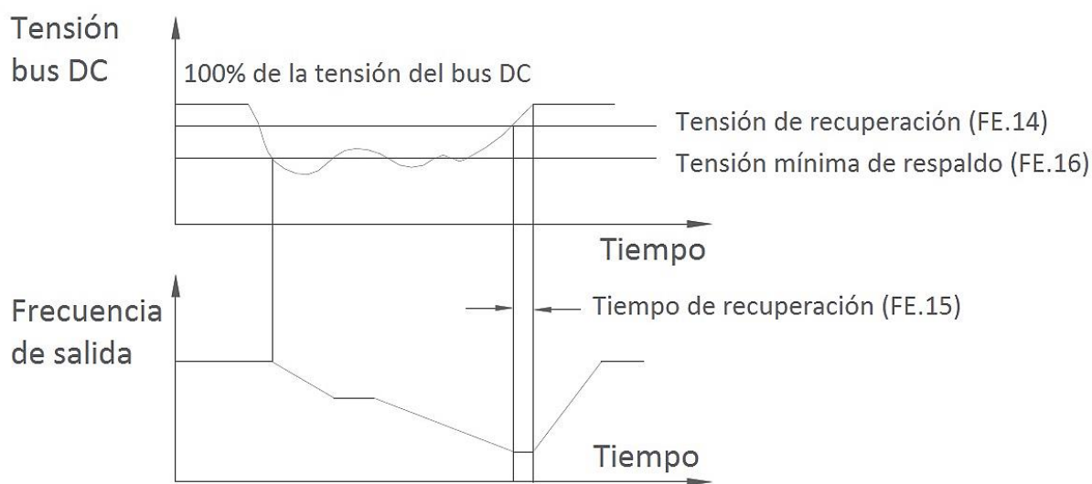
Figura 6-12-1 Función de respaldo
