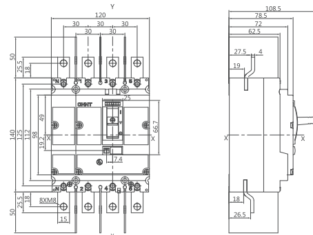
Diagram 1. NM8N(DC, SD)-125
